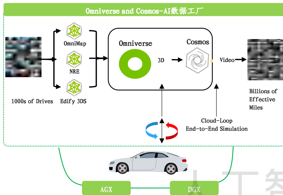
智能驾驶三类计算系统
