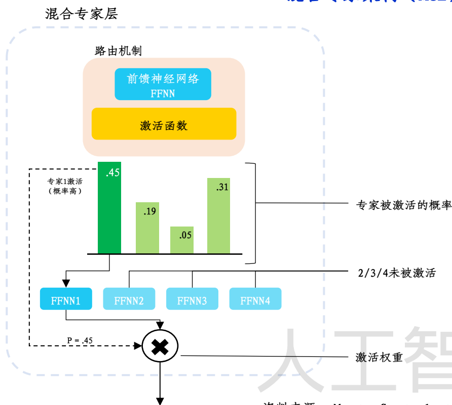
混合专家架构（MoE）原理图
