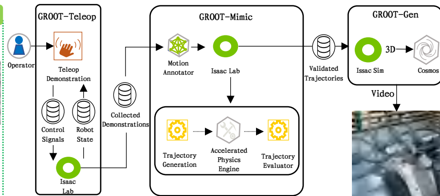
Isaac GROOT运动合成系统
