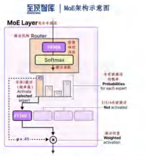
MoE架构示意图
